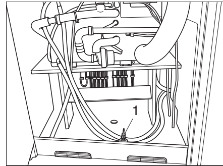
Kuva 122 Poistohanojen sijainti
