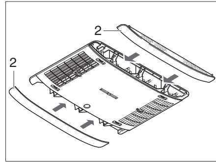
Kuva 157 Paneelit ilmastointilaite
