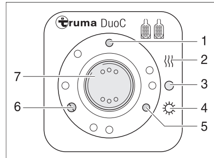
Kuva 86 Säätyksikkö
