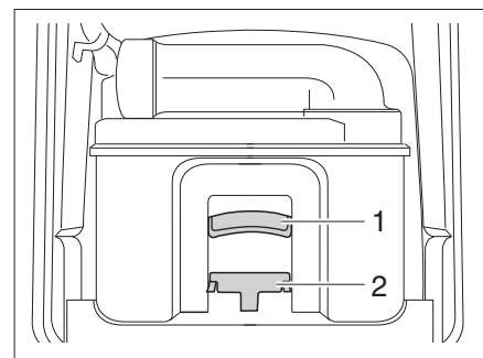
Kuva 146 Thetford-kasetti
